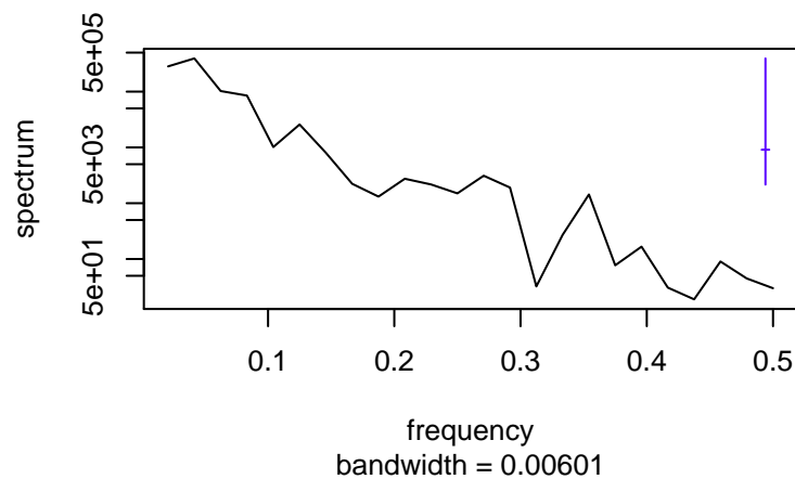
Trend
