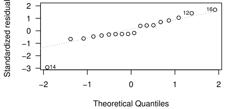
Normal Q-Q
