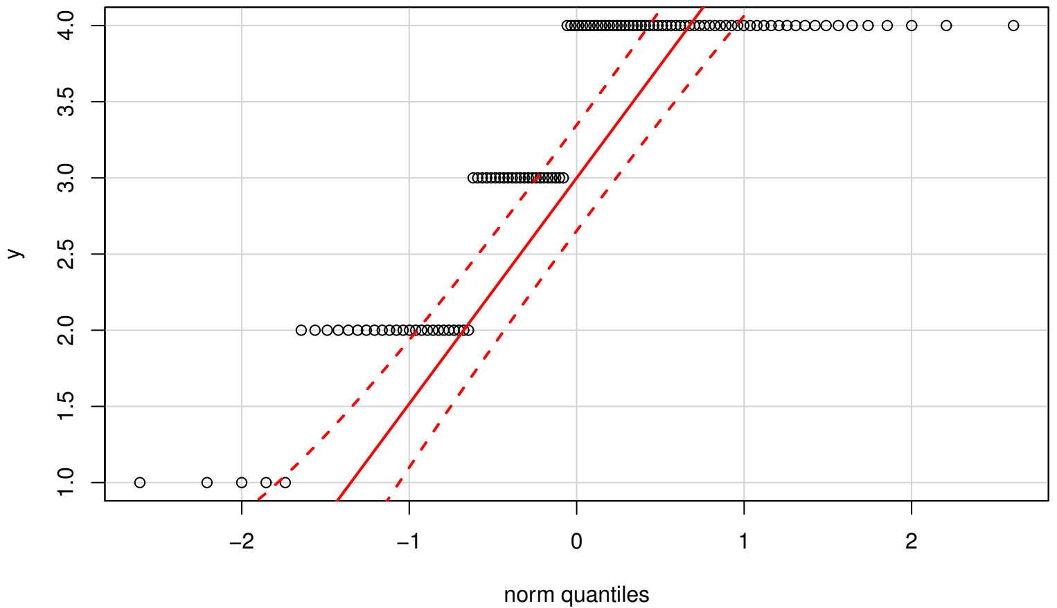
QQplot of variable y
