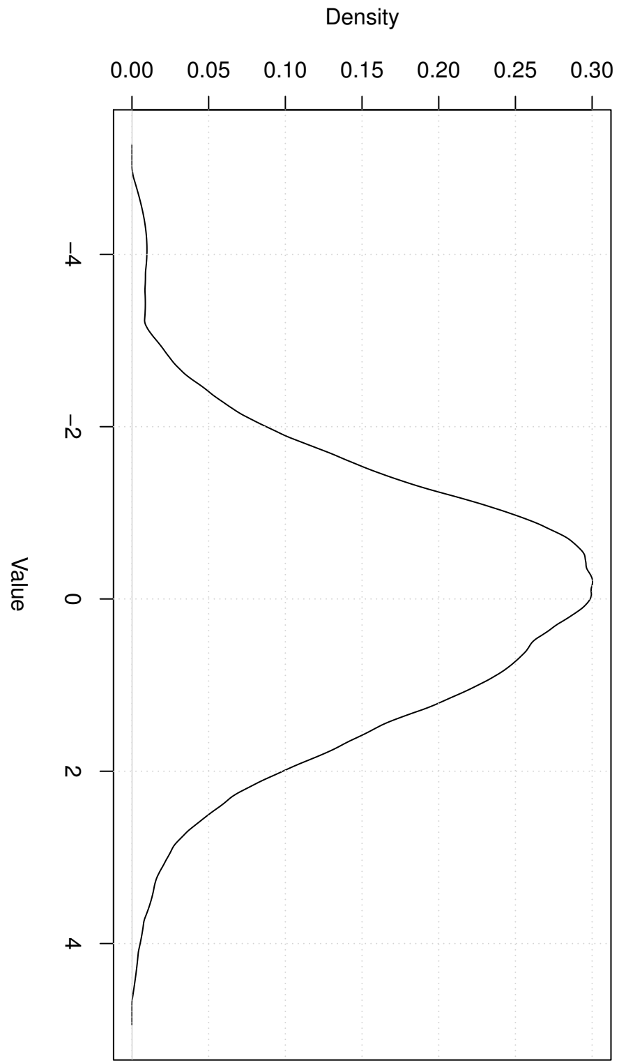
Optcosine Kernel
