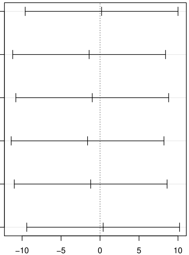
Differences in mean levels of GeslachtLabel:GroepLabel
