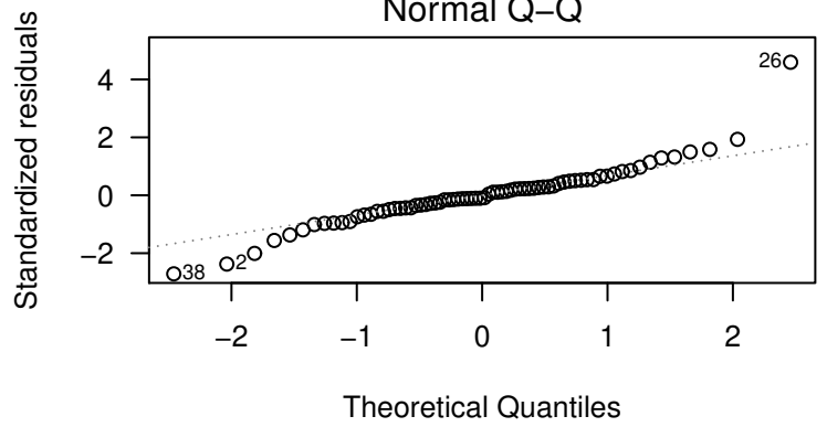
Normal Q-Q
