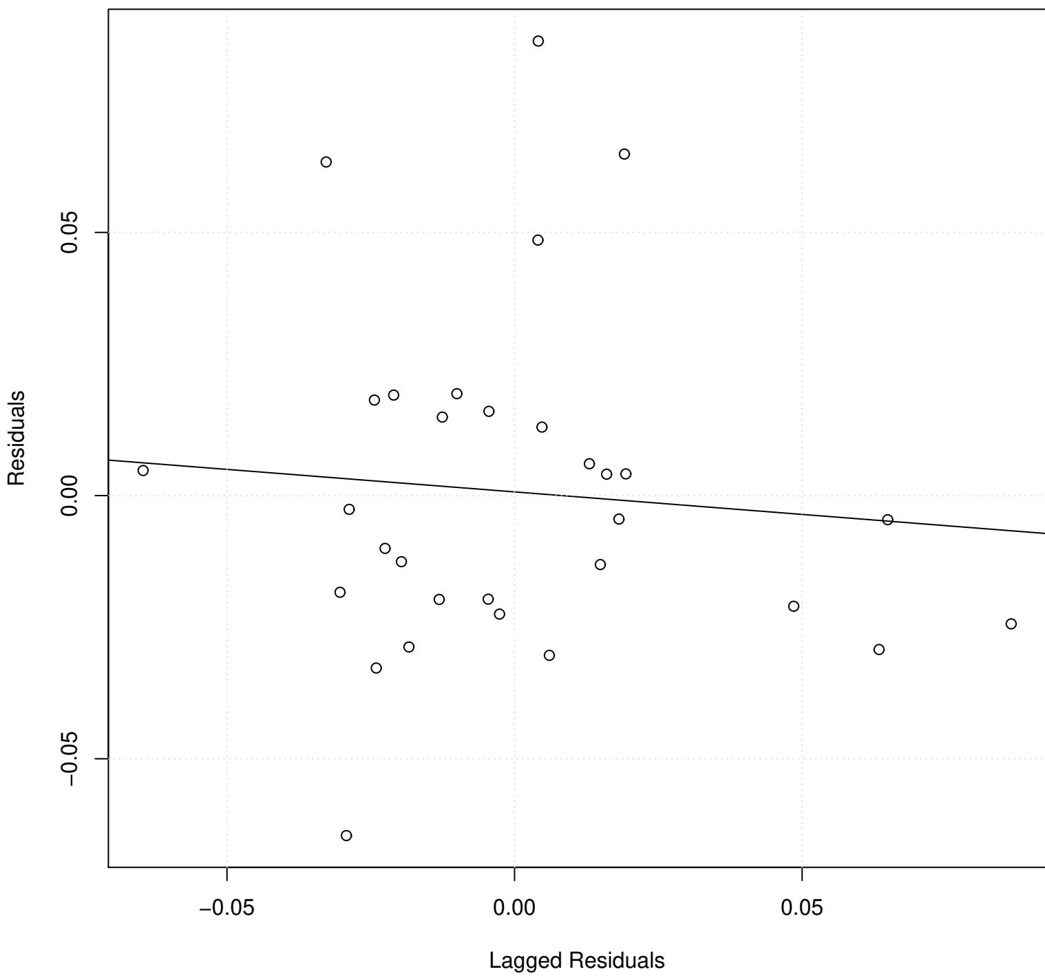
Lag plot
