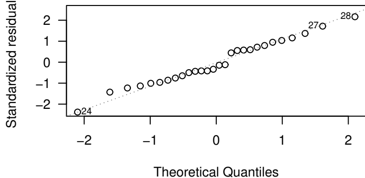
Normal Q-Q
